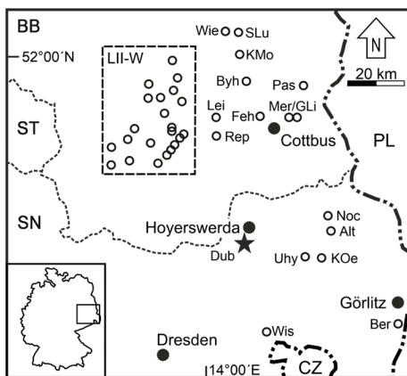
Abb. 1: Lage des Dubringer Moores bei Hoyerswerda (Dub) mit Darstellung anderer palynologisch untersuchter Lokalitäten in Südost-Brandenburg und Nordost-Sachsen (erweitert aus DE KLERK & JOOSTEN 2016). Alt: Altliebel (WARMBRUNN 1999, KÜSTER & WARMBRUNN 2000) und Großteich Altliebel/Reichswalde (FRIEDRICH et al. 2001); Ber: Moor bei Berzdorf (MÜLLER 1968); Byh: Byhleguhrer Bagen (STRAHL 2005); Feh: Fehrow (BRANDE et al. 2007); GLi: Düne bei Groß Lieskow (BITTMANN & PASDA 1999); KMo: Kleiner Mochowsee (JAHNS 1999); KOe: Klein Oelsa (WARMBRUNN 1999, KÜSTER & WARMBRUNN 2000); Lei: Leipe (BRANDE et al. 2007); LII-W: Gebiet mit insgesamt 22 pollenanalytisch untersuchten Lokalitäten (LANGE et al. 1978); Mer: Merzdorf 31 (JAHNS 2004), und Merzdorf 31, Profile 1–5 (POPPSCHÖTZ & STRAHL 2004); Noc: Nochten (DINIES 2021); Pas: Pastlingsee (JAHNS et al. 2013); Rep: CRep 89/2 (DE KLERK 2004); SLu: Sawaller Luch (STRAHL 2013); Uhy: Uhyest CUH 86/1 (KLOSS 1991; DE KLERK 2005); Wie: Wiese (ILLIG & LANGE 1992); Wis: Wiesen (MÜLLER 1968). BB: Brandenburg; ST: Sachsen-Anhalt; SN: Sachsen; PL: Polen; CZ: Tschechische Republik.
